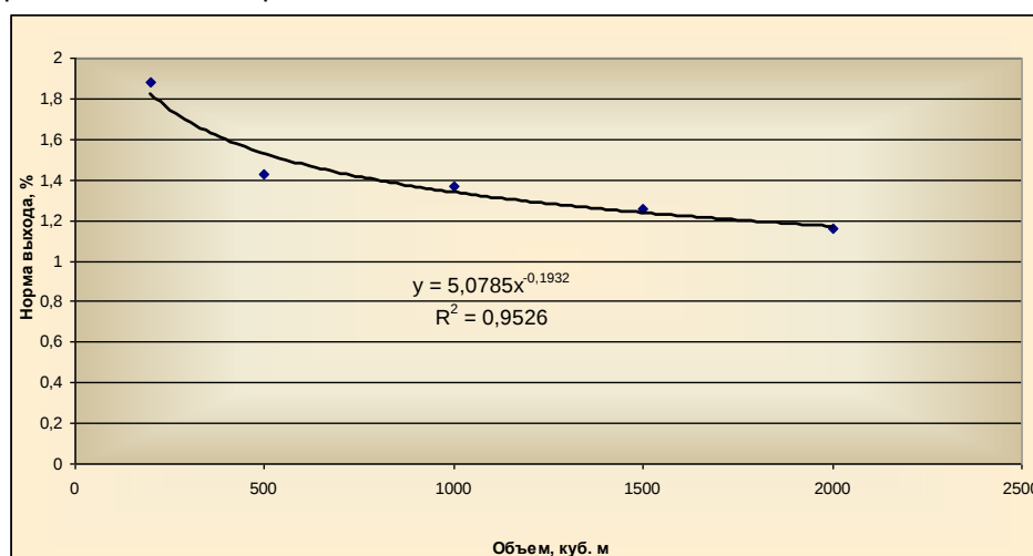
Рис. 12. Зависимость нормы выхода годных материалов для шифра 2-1-4
